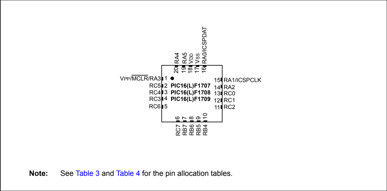
PIN DIAGRAM – 20-PIN QFN
