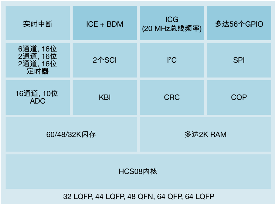
AC60结构框图
